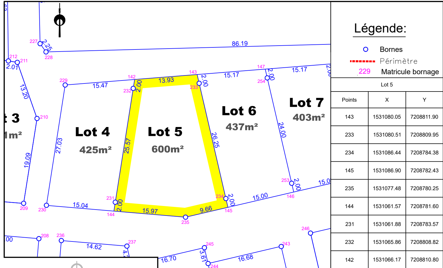
PLAN DE DÉLIMITATION- Echelle: 1/500
